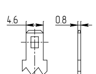
Клемма F1А
