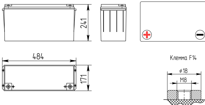
Расположение клемм D
